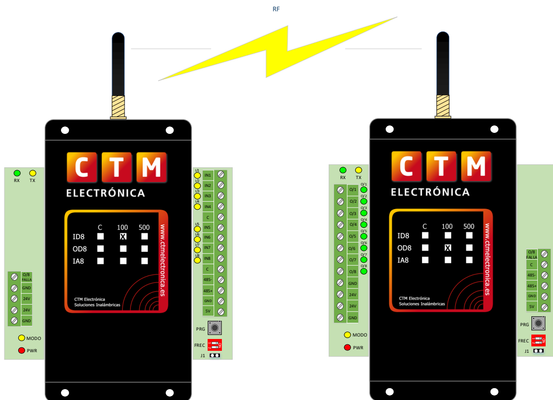
Ejemplo típico de conexionado de un sistema punto a punto de 16 entradas/16 salidas
